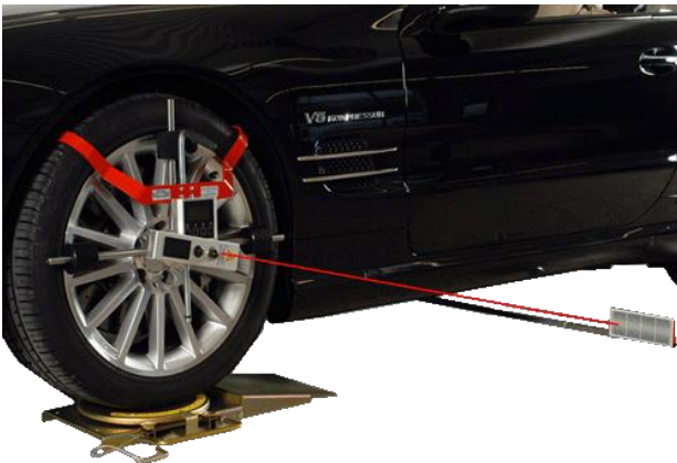
Vue d'ensemble du kit MT-HD-10, système contrôle train avant / arrière
