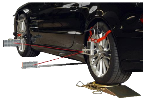
Vue d'ensemble du kit MT-HD-10, système contrôle train avant / arrière
