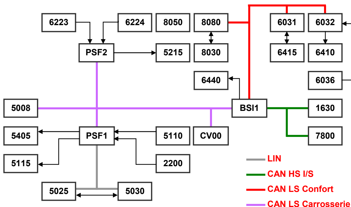
SCHEMA « FONCTION VISIBILITE »
