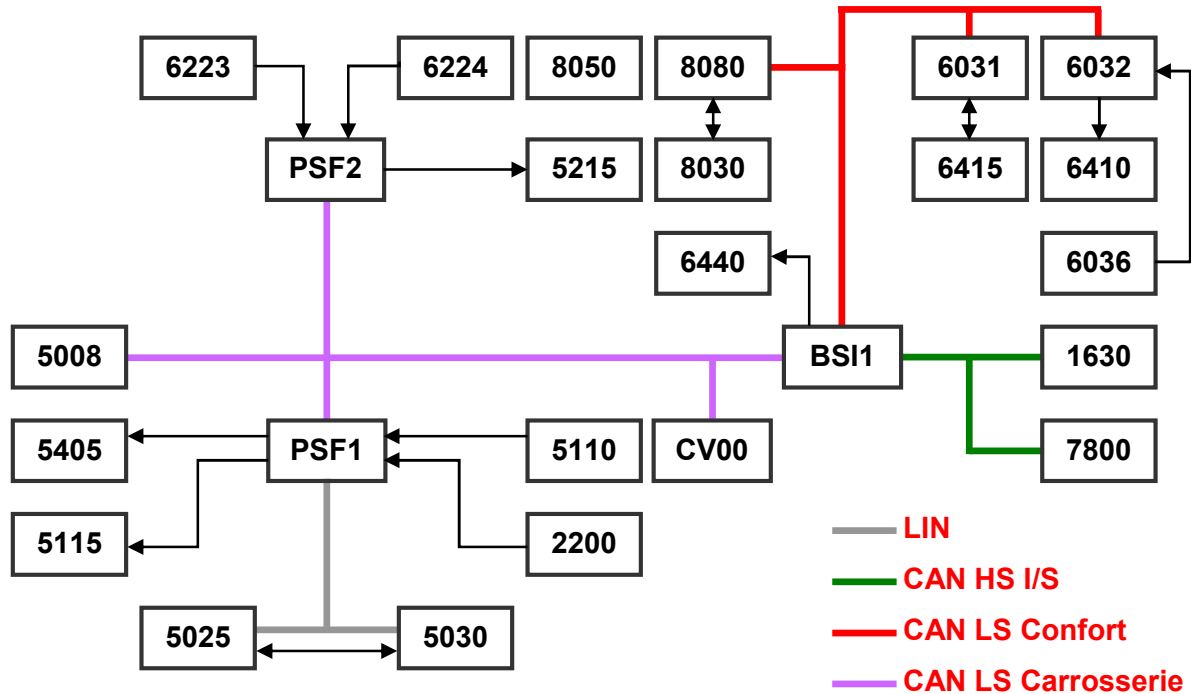
SCHEMA DES RESEAUX MULTIPLEXES
